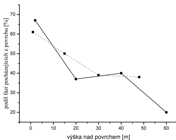
Obr. 2. Procentuální zastoupení půdních minerálů z celkového počtu nalezených minerálů (viz text). Plnou čarou je označen profil z Kopist, tečkovanou profil z Dlouhé Louky
